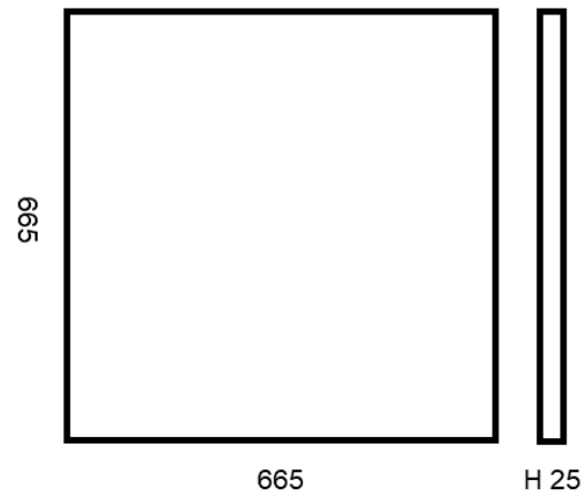
Einbaurahmen M
